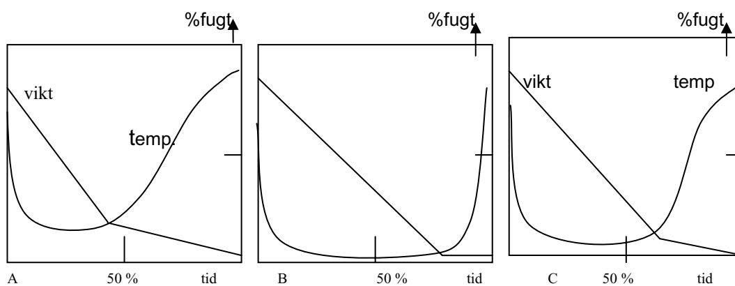
Figur 3 Generelle skitser over tørringsforløb A, B og C
